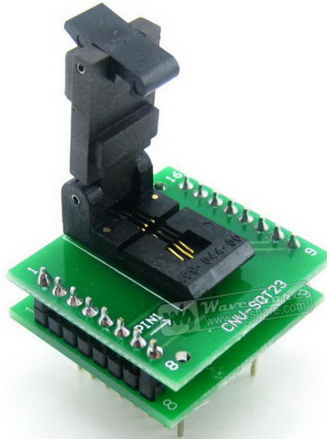
2. Ilustrace: Programovací patice pro SOT23-6
